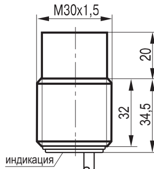
Габаритный чертеж
